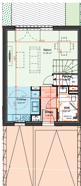
0. RDC 1:125
